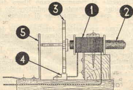
Fig. 4 - Il complesso montato visto di fianco.
