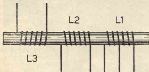
Fig. 2 - Bobine L1 - L2 - L3 avvolte su nucleo ferroxcube.
