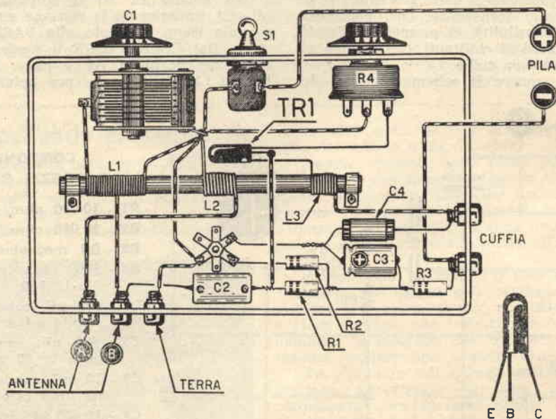
Fig. 3 - Schema pratico.
