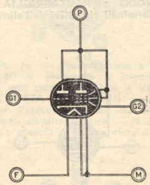
Fig. 8. — Trovandosi nella necessità di collaudare un tipo di valvola non considerato in tabella, in figura viene indicato il modo di collegare gli elettrodi di una valvola PEN-TODO-TRIODO ai terminali rispettivi dell'alimentatore. Come è possibile notare, del tipo di valvola considerato si possono sottoporre a collaudo le due sezioni, inserendo la griglia (G1 e G2) ai rispettivi terminali dell'alimentatore G1 e G2).
