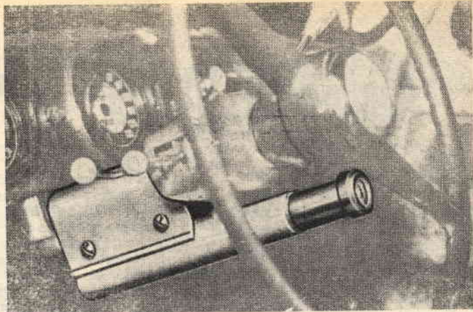
Fig. 3. — BRANC antifurto fermasterzo con allarme acustico per tutti i modelli di vetture FIAT.
