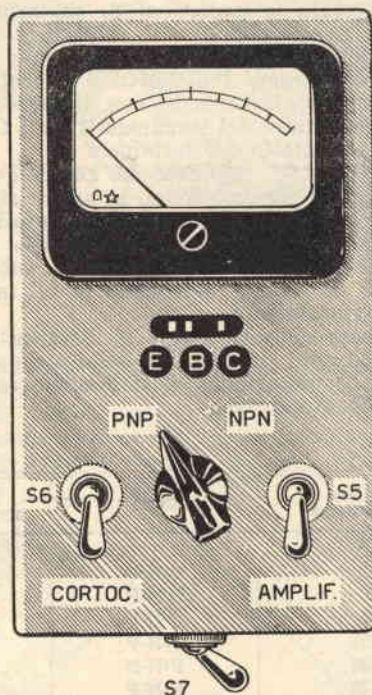
Fig. 3 - Pannello frontale del prova-transistori.
