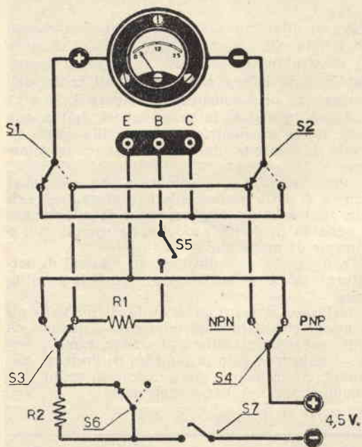
Fig. 1 - Schema elettrico del prova-transistori.
