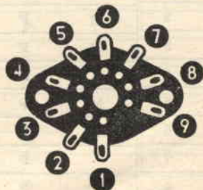
Fig. 16. — Numerazione progressiva assegnata ai piedini di uno zoccolo tipo NOVAL (vedi tabella n. 1) per l'esecuzione dei collegamenti all'alimentatore. — N. B. - Lo zoccolo s'intende visto dal disotto.
