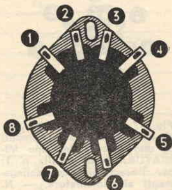
Fig. 15. — Numerazione progressiva assegnata ai piedini di uno zoccolo del tipo a VASCHETTA (vedi tabella n. 1) per l'esecuzione dei collegamenti all'alimentatore. — N. B. - Lo zoccolo s'intende visto dal disotto.
