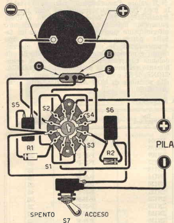
Fig. 2 - Schema pratico del prova-transistori.
