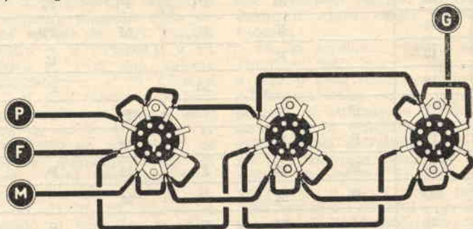
Fig. 18. — Così si presentano i collegamenti dei primi tre zoccoli (3 - 2 - 1) tipo OCTAL nel nostro provavalvole, visto, ben s'intende, dal disotto.
