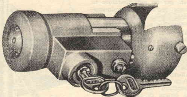
Fig. 1. — ANTIFURTO B.S.O. (bloccasterzo O.M.C.A.) con allarme acustico per FIAT 600.
