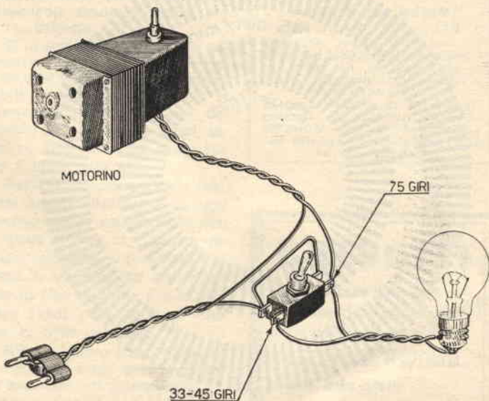
Fig. 2 - Schema pratico dell'applicazione. Per l'inserimento o il disinserimento della lampada si è ricorsi all'ausilio di un deviatore a levetta.
