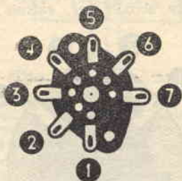
Fig. 17. — Numerazione pro- gressiva assegnata ai piedini di uno zoccolo del tipo MI- NIATURA (vedi tabella n. 1) per l'esecuzione dei collega- menti all'alimentatore. — N. B. - Lo zoccolo s'intende visto dal disotto
