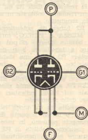
Fig. 12. — Trovandosi nella necessità di collaudare un tipo di valvola non contemplato in tabella, viene indicato in figura il modo di collegare gli elettrodi di un doppio TRIDO ai rispettivi terminali dell'alimentatore. Pure per detto tipo di valvola è possibile la prova separata delle due sezioni.
