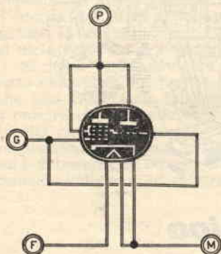
Fig. 9. — Essendo nella necessità di sottoporre a collaudo un tipo di valvola non contemplato in tabella, viene indicato a figura il metodo di collegamento degli elettrodi di una valvola convertitrice EP-TODO o PENTAGRIGLIA ai terminali rispettivi dell'alimentatore.
