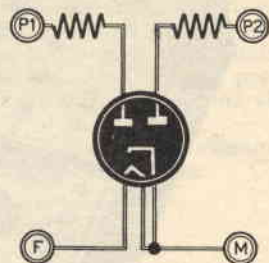
Fig. 11. — Essendo nella necessità di sottoporre a collaudo un tipo di valvola non contemplato in tabella, viene indicato a figura il metodo di collegamento degli elettrodi di una valvola raddrizzatrice ai rispettivi terminali; dell'alimentatore. Si noti come, in serie alle due sezioni delle placche, risultino inserite due resistenze, il cui valore dovrà essere ricercato sperimentalmente ad impedire che la lancetta dello strumento si porti a fondo scala.
