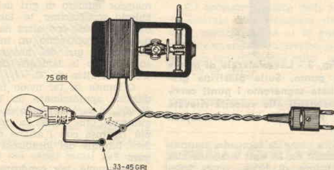
Fig. 1 - Per ridurre la velocità di un motorino da 78 a 45 giri sarà sufficiente inserire in serie al medesimo una lampada della potenza di 20-25-30 watt.
