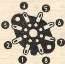
Fig. 14. — Numerazione progressiva assegnata ai piedini di uno zoccolo tipo RIMLOK (vedi tabella n. 1) per l'esecuzione dei collegamenti all'alimentatore. — N. B. - Lo zoccolo s'intende visto dal disotto.
