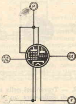
Fig. 10. — Trovandosi nella necessità di collaudare un tipo di valvola non contemplato in tabella, viene indicato a figura il modo di collegare gli elettrodi di una valvola ESODO-TRIDO o EPTODO-TRIDO ai rispettivi terminali dell'alimentatore. Risultando in questo tipo di valvola le due sezioni indipendenti, sarà possibile procedere al collaudo separato del triodo o dell'eptodo.
