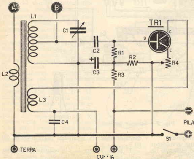
Fig. 1 - Schema elettrico.
