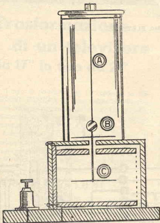
Fig. 1 - Sezione laterale dell'istrumento completato.
