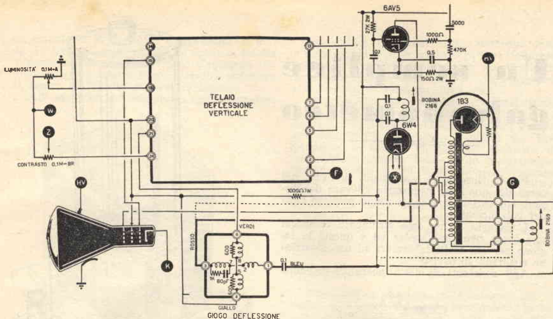
Fig. 1. - SCHEMA ELETTRICO.
