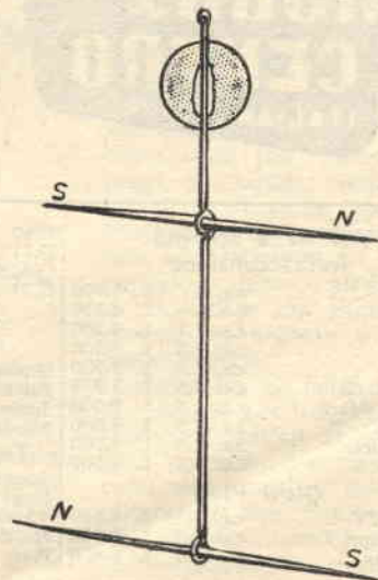
Fig. 4 - Complesso aghi magnetizzati. Si noti l'inversione delle polarità degli aghi stessi.
