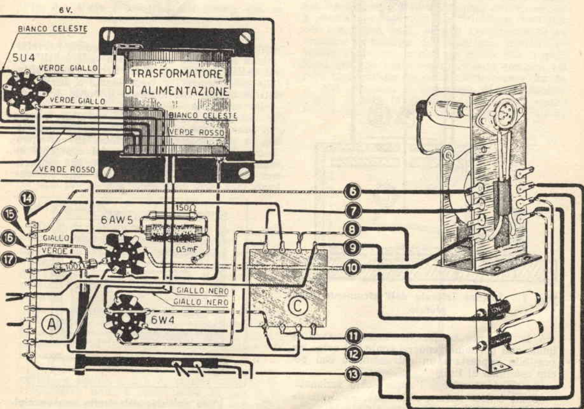
Fig. 2. - SCHEMA PRATICO.
