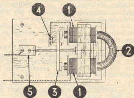
Fig. 5 - Il complesso montato visto in pianta.
